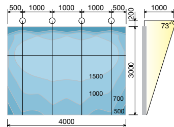
HCF0723BHE + CMT150/WW 13500 lm
