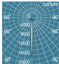
HCF1521BHE + CMT150/WW 13500 lm
