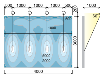
HCF0721BHE + CMT150/WW 13500 lm
