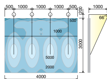
HCF1521BHE + CMT150/WW 13500 lm
