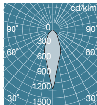
HCF0723BHE + CMT150/WW 13500 lm
