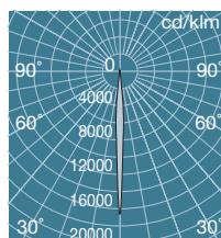
HCF0721BHE + CMT150/WW 13500 lm
